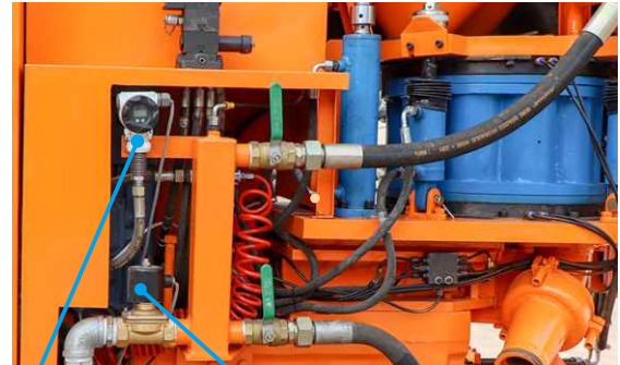
压力传感器
